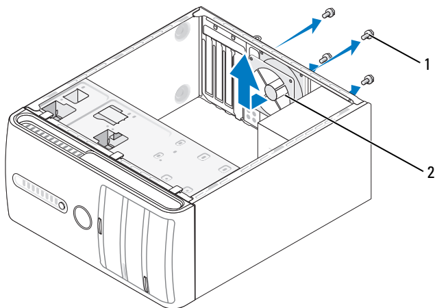
1 螺钉 (4) 2 机箱风扇
