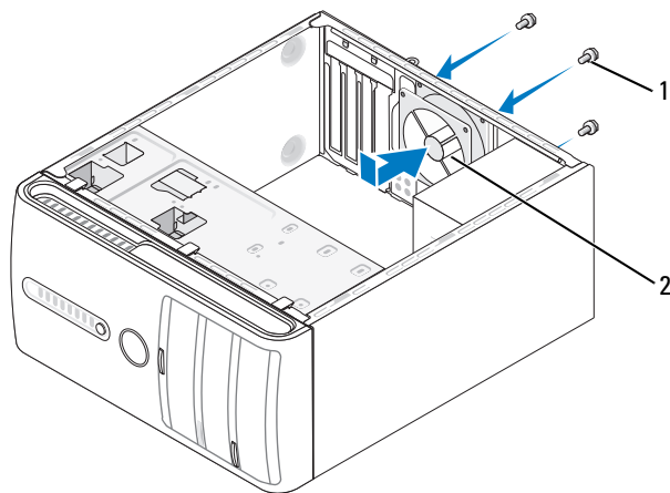
1 螺钉 (4) 2 机箱风扇
