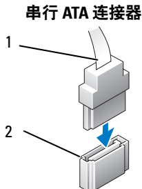
1 接口电缆 2 接口连接器
